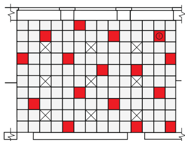
План подвесного потолка (армстронг 600x600 мм) с ориентировочным расположением светильников
